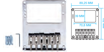
PONTE HUMBUCKER PARA TELE Cód: CGBT-3H CR 6 Saddles fundidos Distanciamento 54mm Travamento das cordas através do corpo
