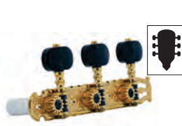
TARRAXA Cód: 35G1600 Dourada knob preto e dourado Par 3L+3R Pino grosso Para violão clássico
