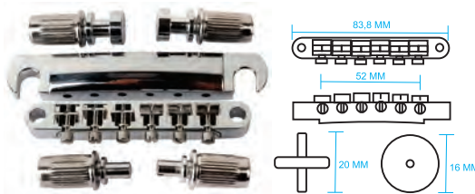
PONTE FIXA LP Cód: CG LP-2 CR Aço
