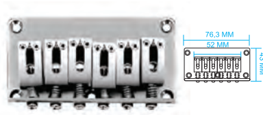
PONTE FIXA HARDTAIL Cód: CGBS-1 6 Saddles fundidos Distanciamento 54mm Travamento das cordas através do corpo
