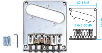
PONTE CROMADA PARA TELE Cód: CGBT-2CR 6 Saddles fundidos Distanciamento 55mm Travamento das cordas através do corpo
