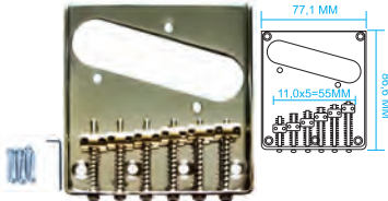
PONTE VINTAGE PARA TELE Cód: CGBT-1 CR 6 Saddles barris Distanciamento 54mm Travamento das cordas através do corpo
