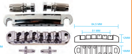
PONTE FIXA LP Cód: CG LP-3 CR Aço
